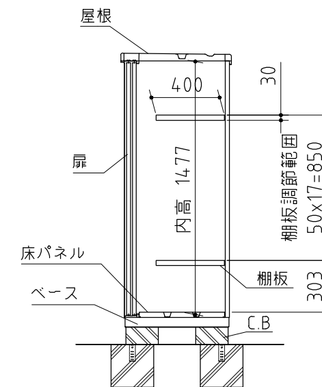
断面図
